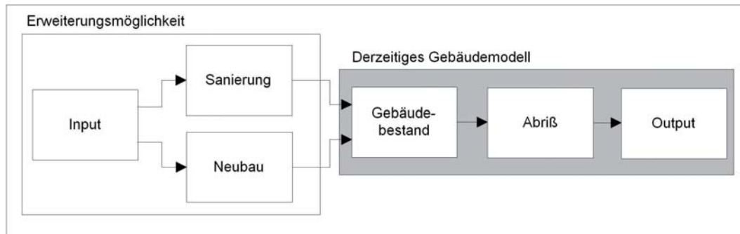
Abb. 7.5 Übersicht über das Gebäudemodell und Erweiterungsmöglichkeiten Dynamisches Gebäudemodell
