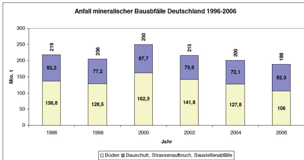
Abb. 7.2 Anfall mineralischer Bauabfälle in Deutschland 1996-2006
