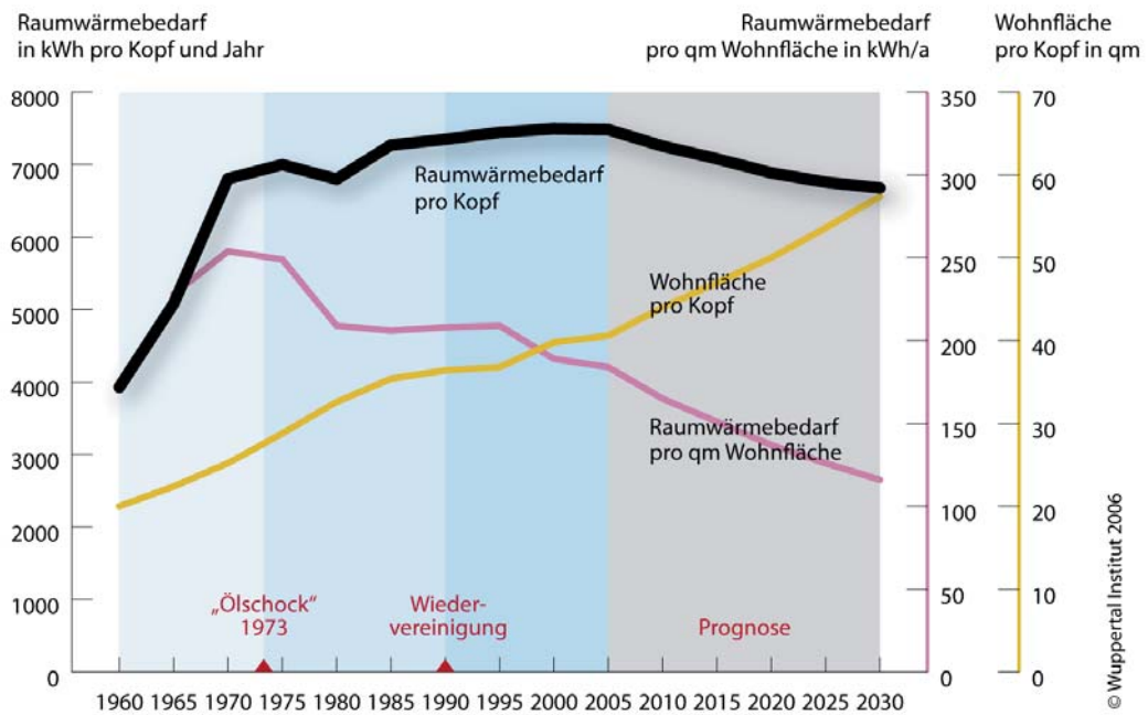
Abb. 6.1 Raumwärmebedarf im Spannungsfeld von Wärmedämmung und Wohnflächennutzung. Raumwärmebedarf ist verstanden als Endenergieverbrauch für Raumwärme ohne Warmwasserbereitung
